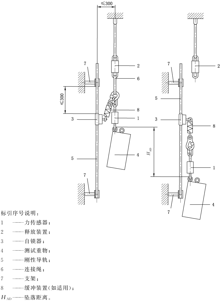
图 5 动态性能测试示意图
